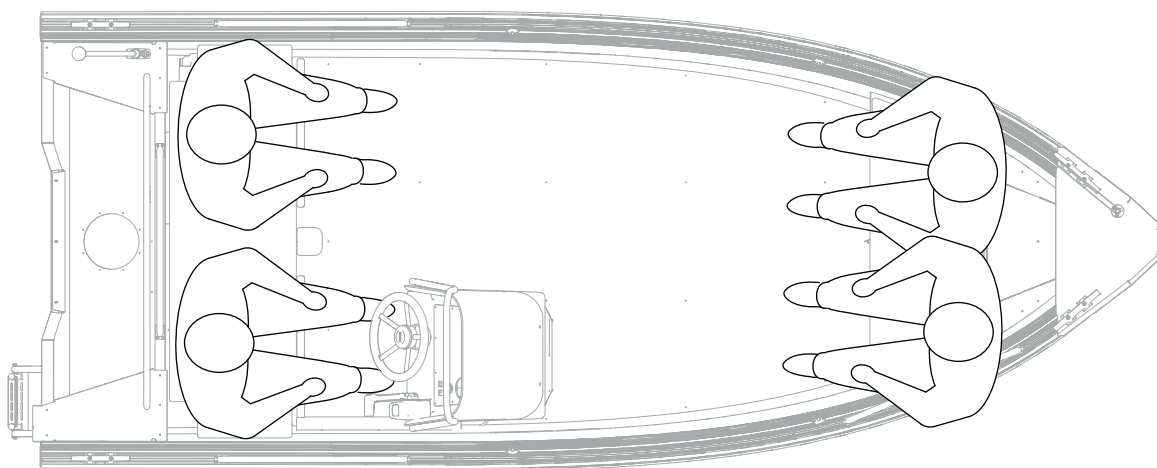
Figur 4.2 Buster S1 seter for maksimalt fire (4) passasjerer
