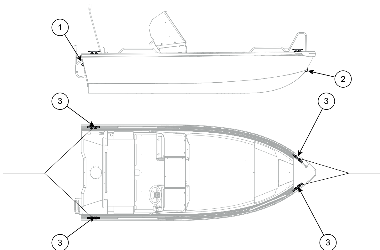
Figur 5.4 Buster S/S1/S2/Scs fortøynings- og slepepunkter
