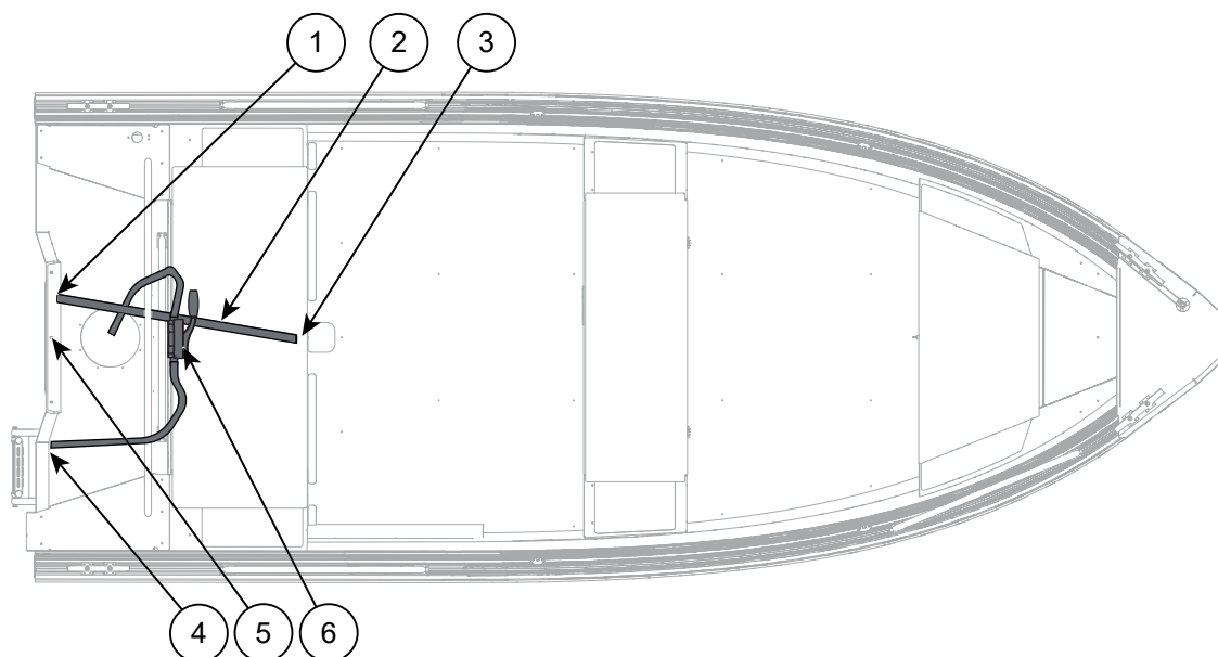
Figur 9.1 Buster S dreneringsutstyrets plasseringer
