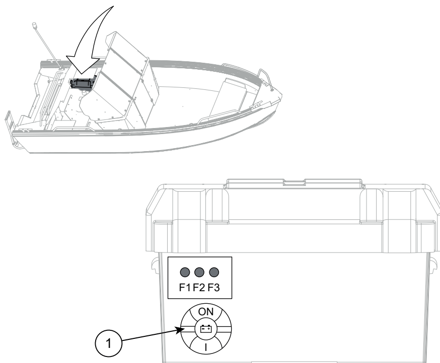
Figur 8.1 Buster S/S1/S2/ScC hovedbryter og sikringspanel
